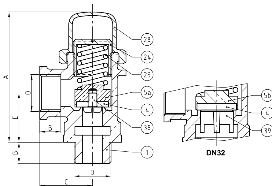
DN15 à 25
