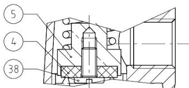
481 / AU481 / 481BP / AU481BP : DN08 à 25
