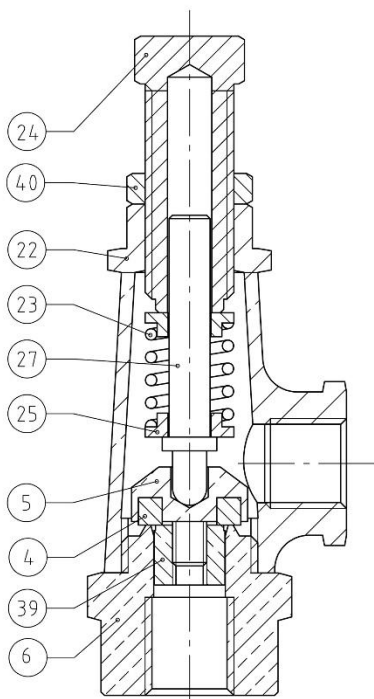
481T / AU481T : DN08 à 15 & 80 481.80 / AU481.80 / 481.80BP / AU481.80BP
