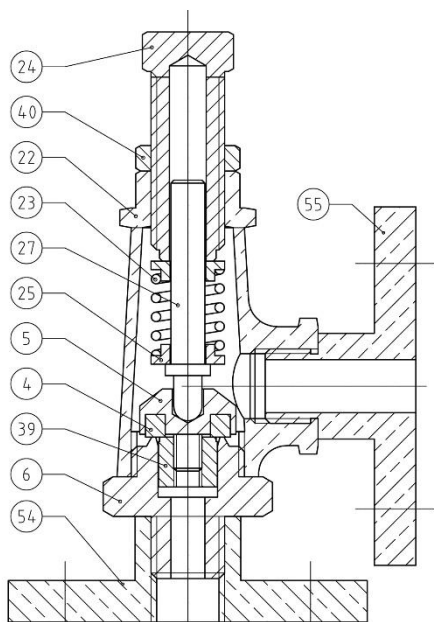
581T / AU581T : DN08 à 15 & 80 581.80 / AU581.80 / 581.80BP / AU581.80BP
