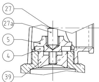
481T / AU481T : DN20 à 65 481 / AU481 / 481BP / AU481BP : DN32 à 65
