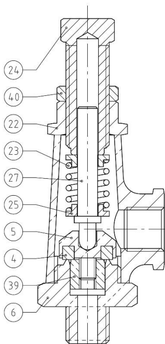
281 / AU281 : DN08 à 15 & 80 381.80 / AU381.80 / 381.80BP / AU381.80BP
