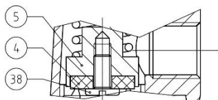
581 / AU581 / 581BP / AU581BP : DN08 à 25
