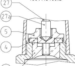
280 / AU280 : DN20 à 65 380 / AU380 / 380BP / AU380BP : DN32 à 65
