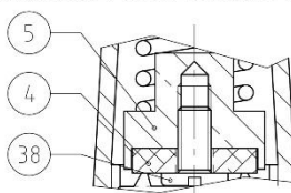
480 / AU480 / 480BP / AU480BP : DN08 à 25
