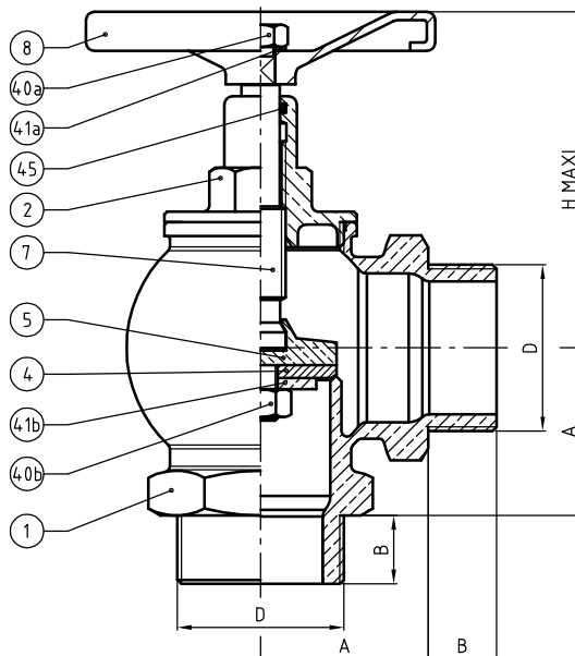
DN40 & DN50
