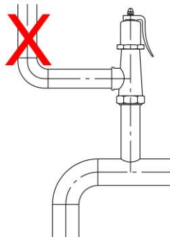
Montage déconseillé
